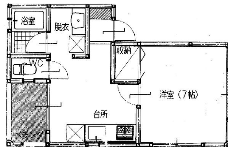
●間取図
